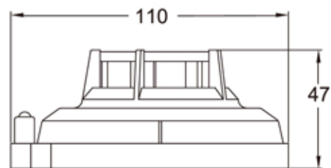
尺寸圖
