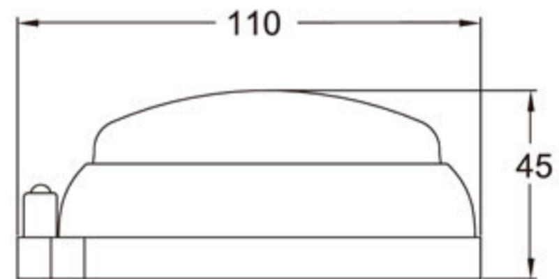
尺寸圖
