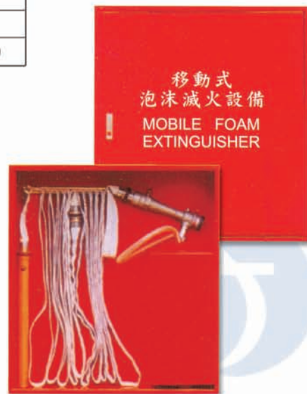
泡沫消防栓箱 HB-F
